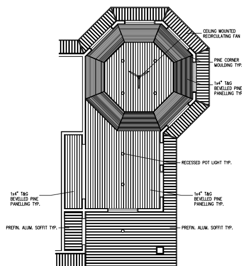
8 Ceiling Plan A-1 Scale: 1/4"=1'
