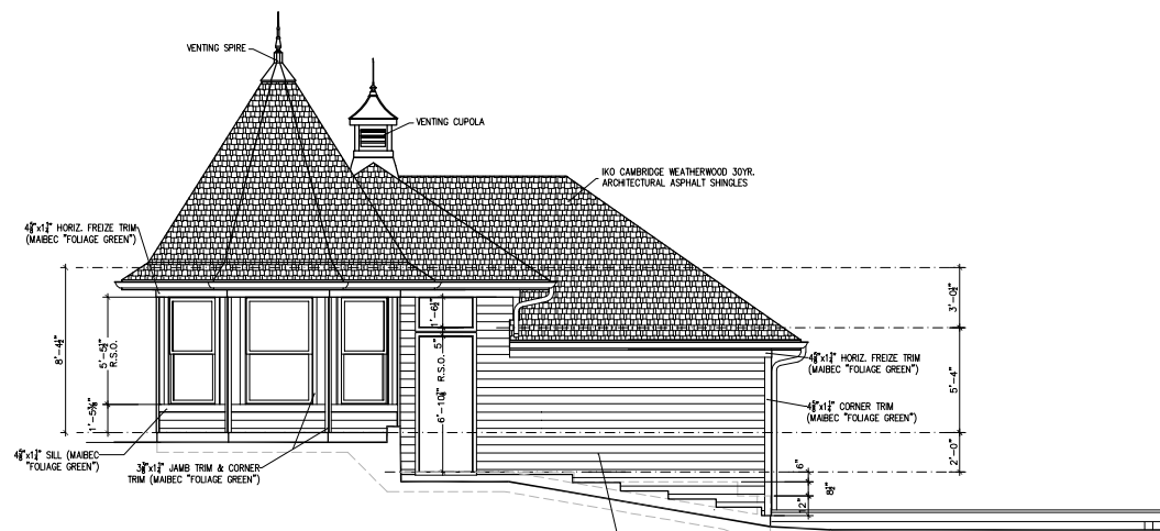
4 West Elevation A-1 Scale: 1/4"=1'
